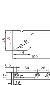
WSPORNIK DOLNY BOTTOM SUPPORT
