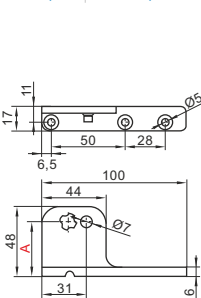
WSPORNIK GÓRNY UPPER SUPPORT
