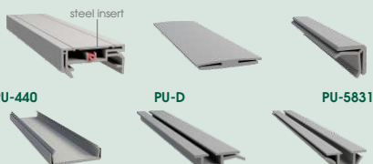
THERMAL BRIDGES IN THE DOOR STRUCTURE MOSTKI CIEPLNE KORPUSU DRZWI
