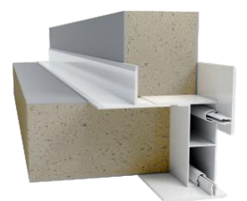
PROFILE DO KOMÓR CHŁODNICZYCH COLD-ROOM PROFILES
