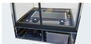
ELEMENTY TERMOFORMOWANE (WANNY IZOLOWANE DO URZĄDZEŃ CHŁODNICZYCH) THERMOFORMED ELEMENTS (INSULATED BASE BOTTOM FOR REFRIGERATED FURNITURE)
